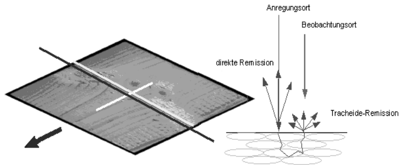
Abb. 3: Erfassen des Tracheide-Effektes (rechts: Querschnitt entlang weißer Linie)
